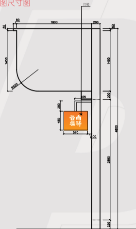
右视图
