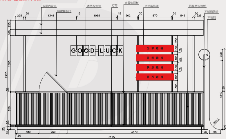
W-4立面图
