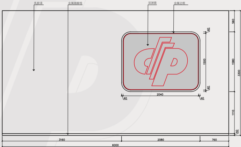
N-1立面图
