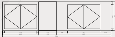
G-2立面图
