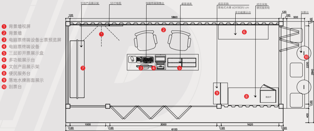
A-1.4 造型比例尺寸规范 平面功能图
