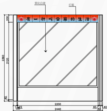
N-3立面图
