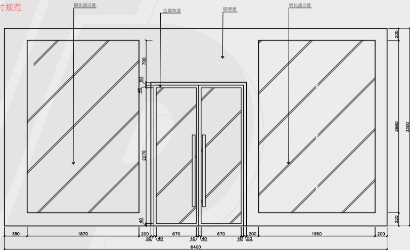
N-4立面图
