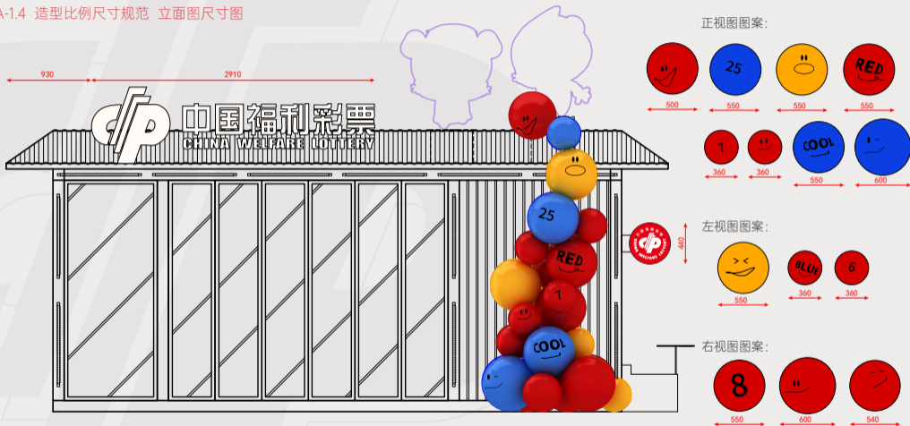
W-1立面图
