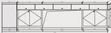
G-3立面图
