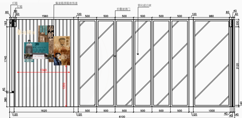
N-4立面图
