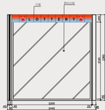
N-2 立面图
