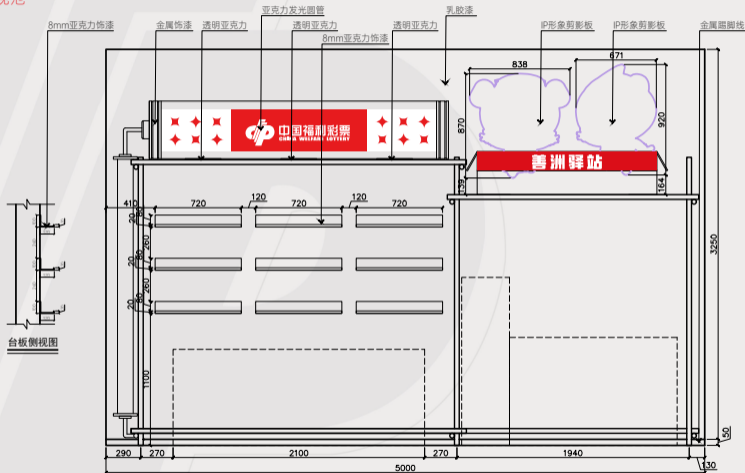
N-2立面图
