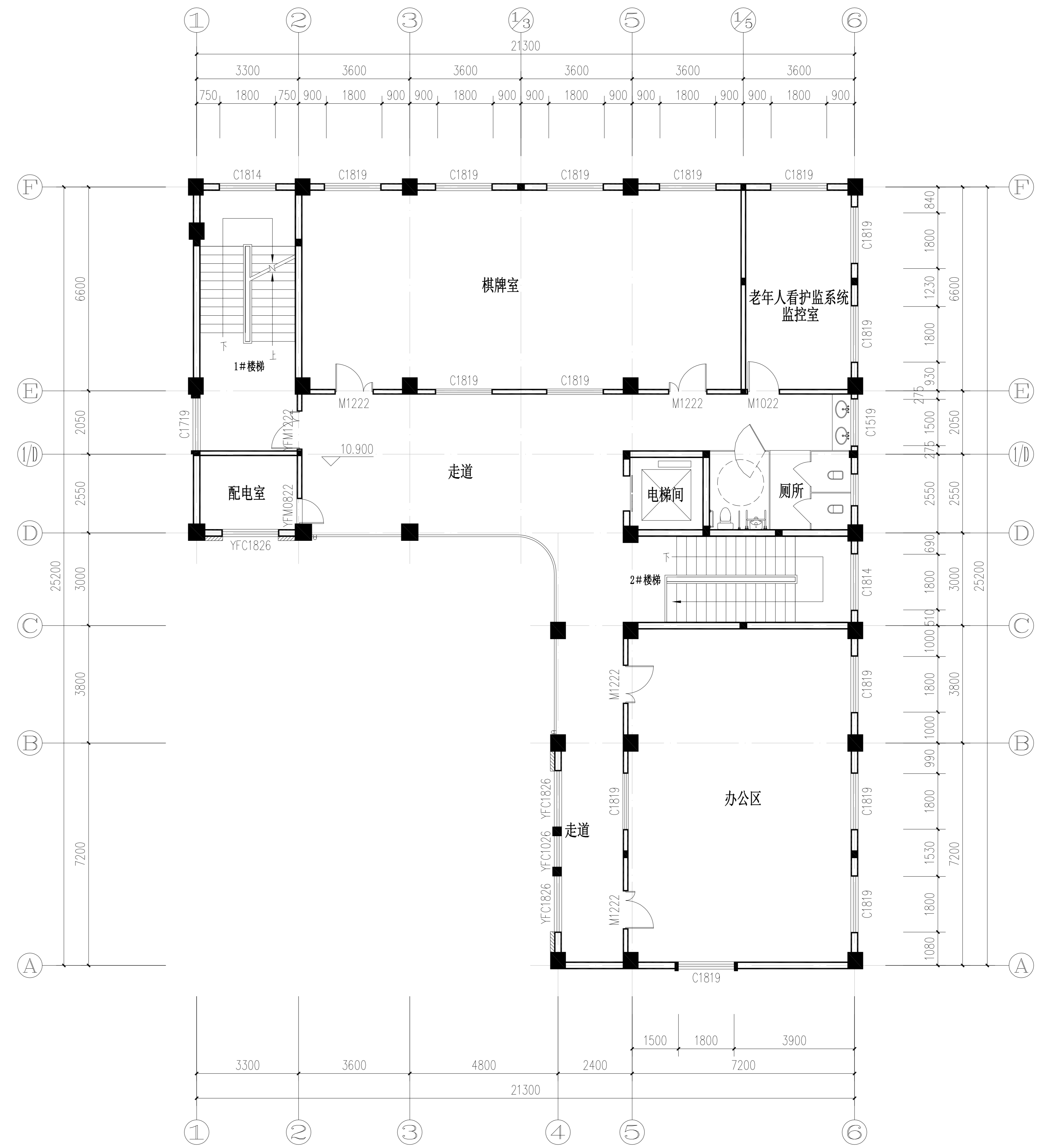
四层平面图 1:100
