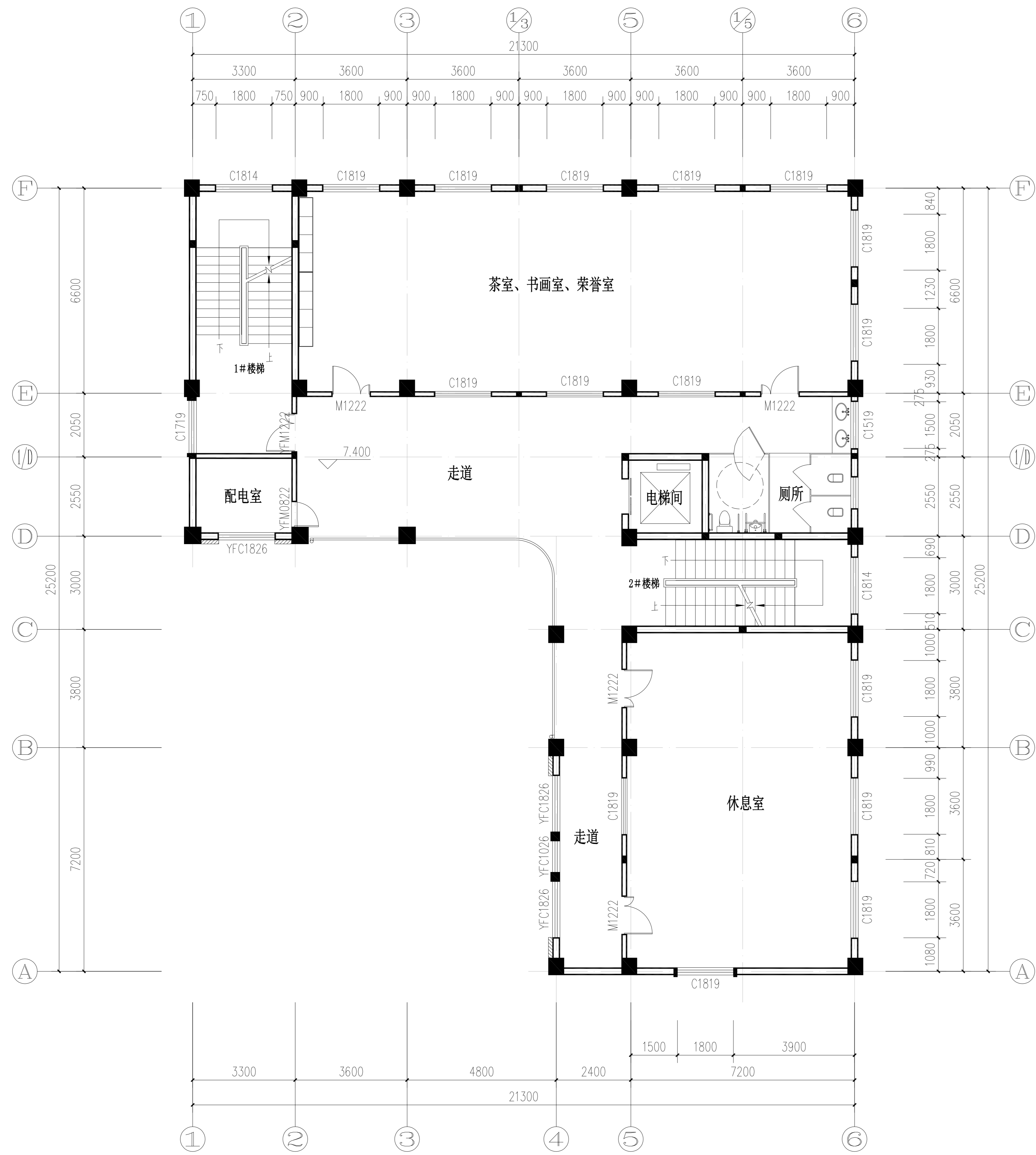
三层平面图 1:100
