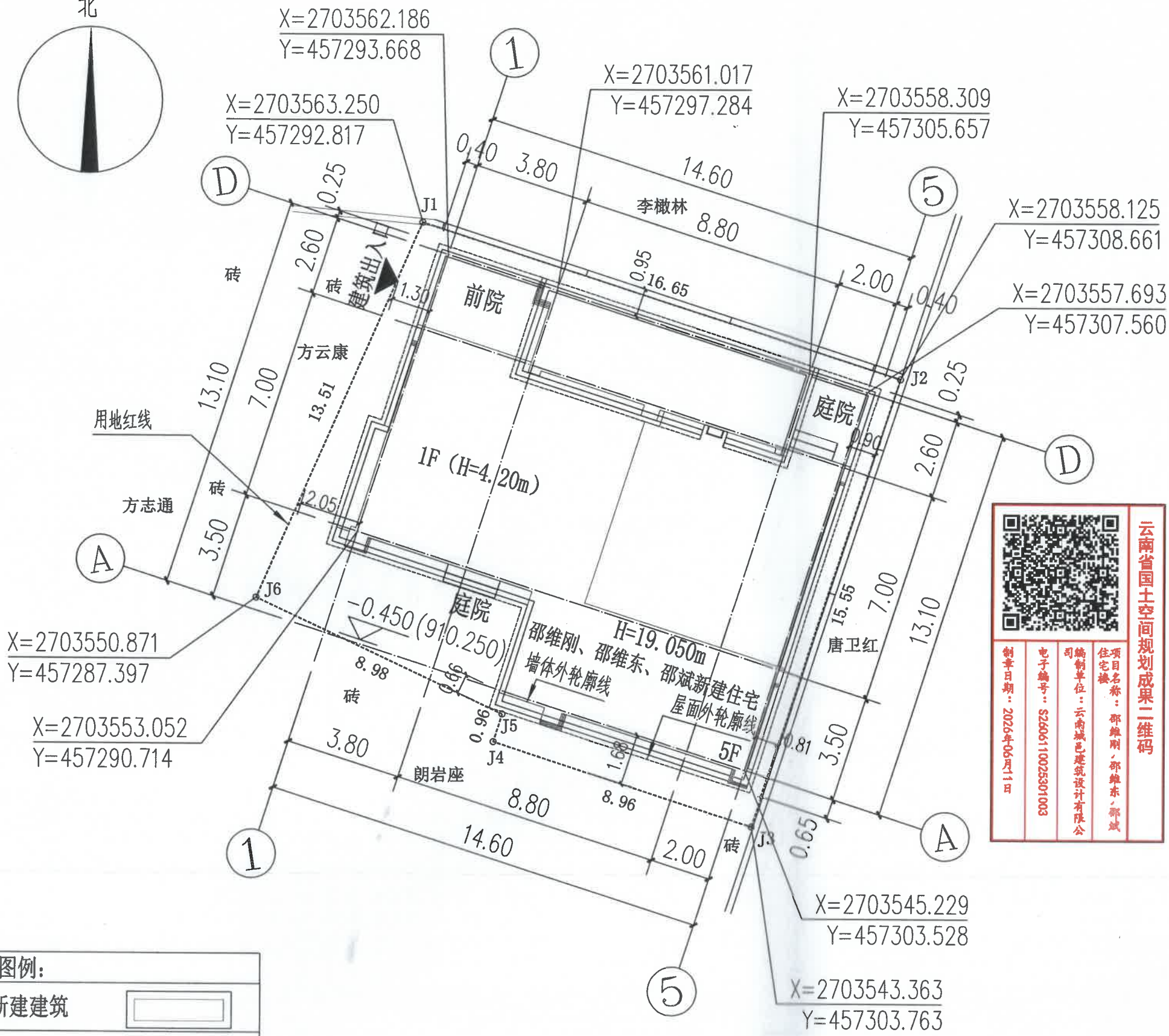
邵维刚、邵维东、邵斌住宅楼总平面布置图 1:200
