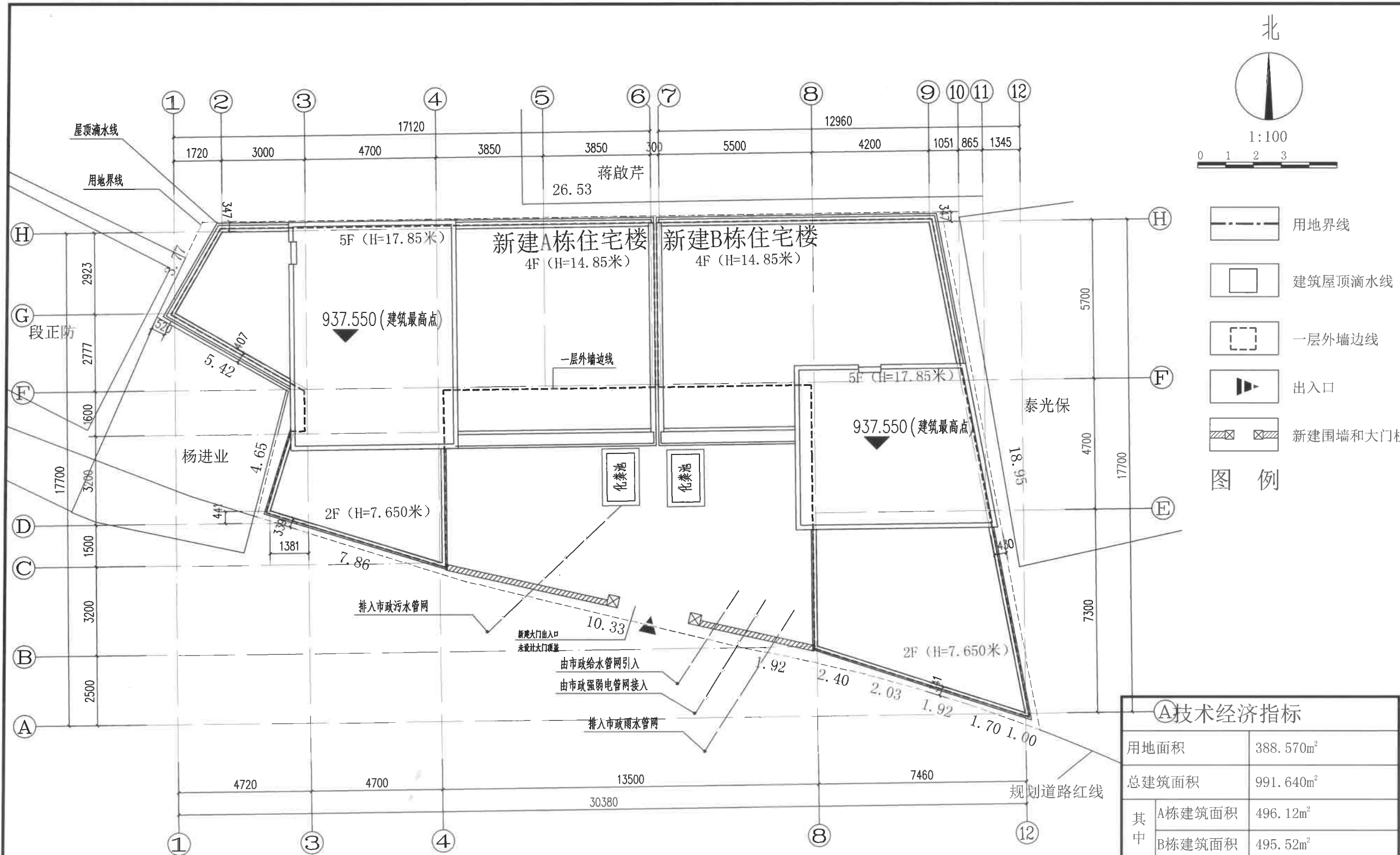
总平面图规划图 1:100 注：图示建筑的尺寸及坐标均为轴线标注。
