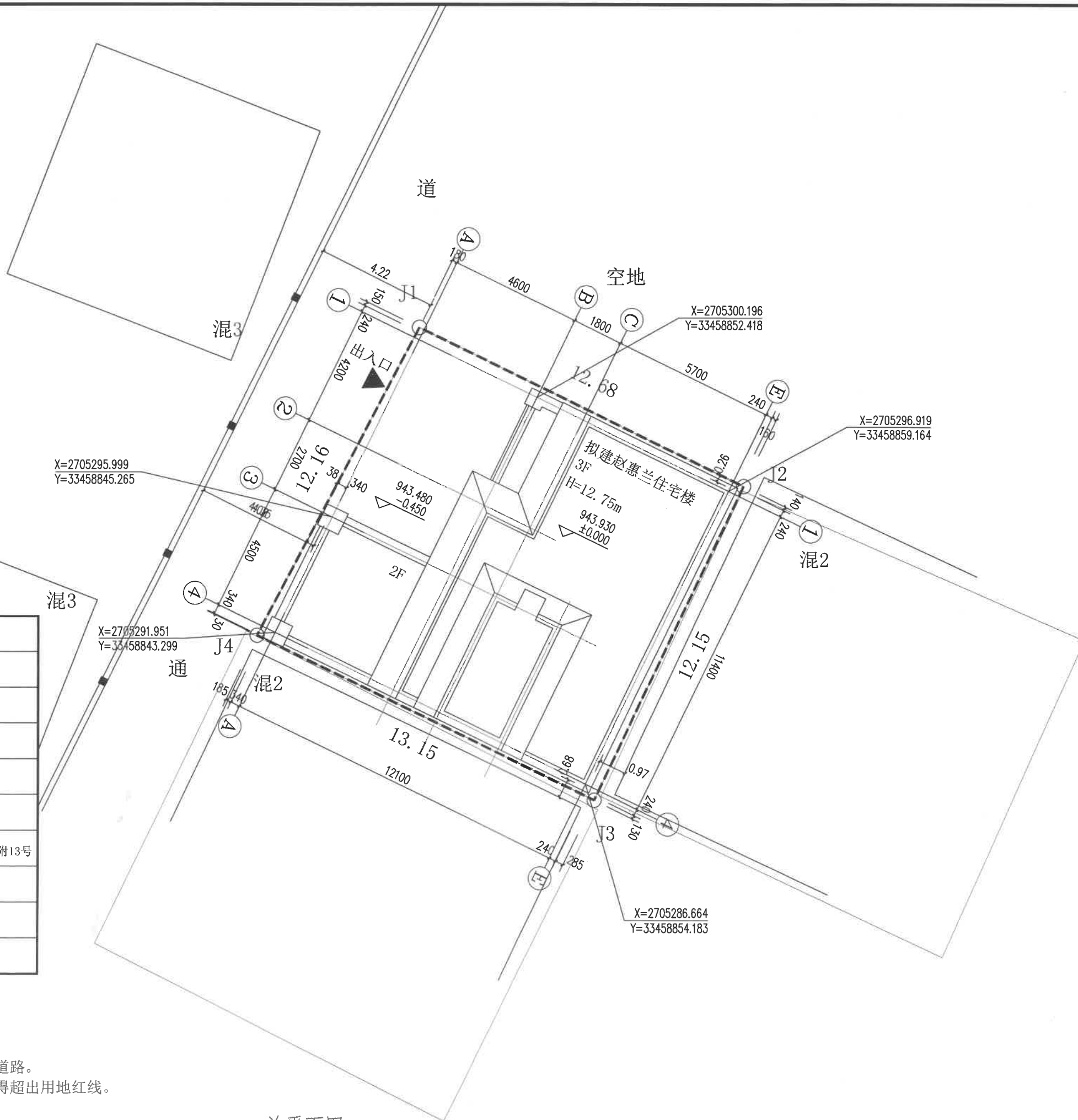
总平面图 1:100
