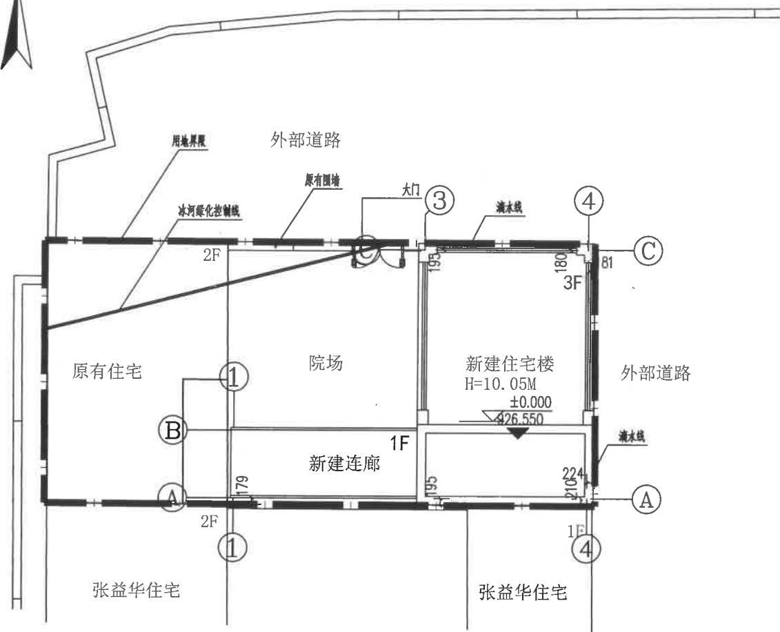
总平面布置图 1:100
